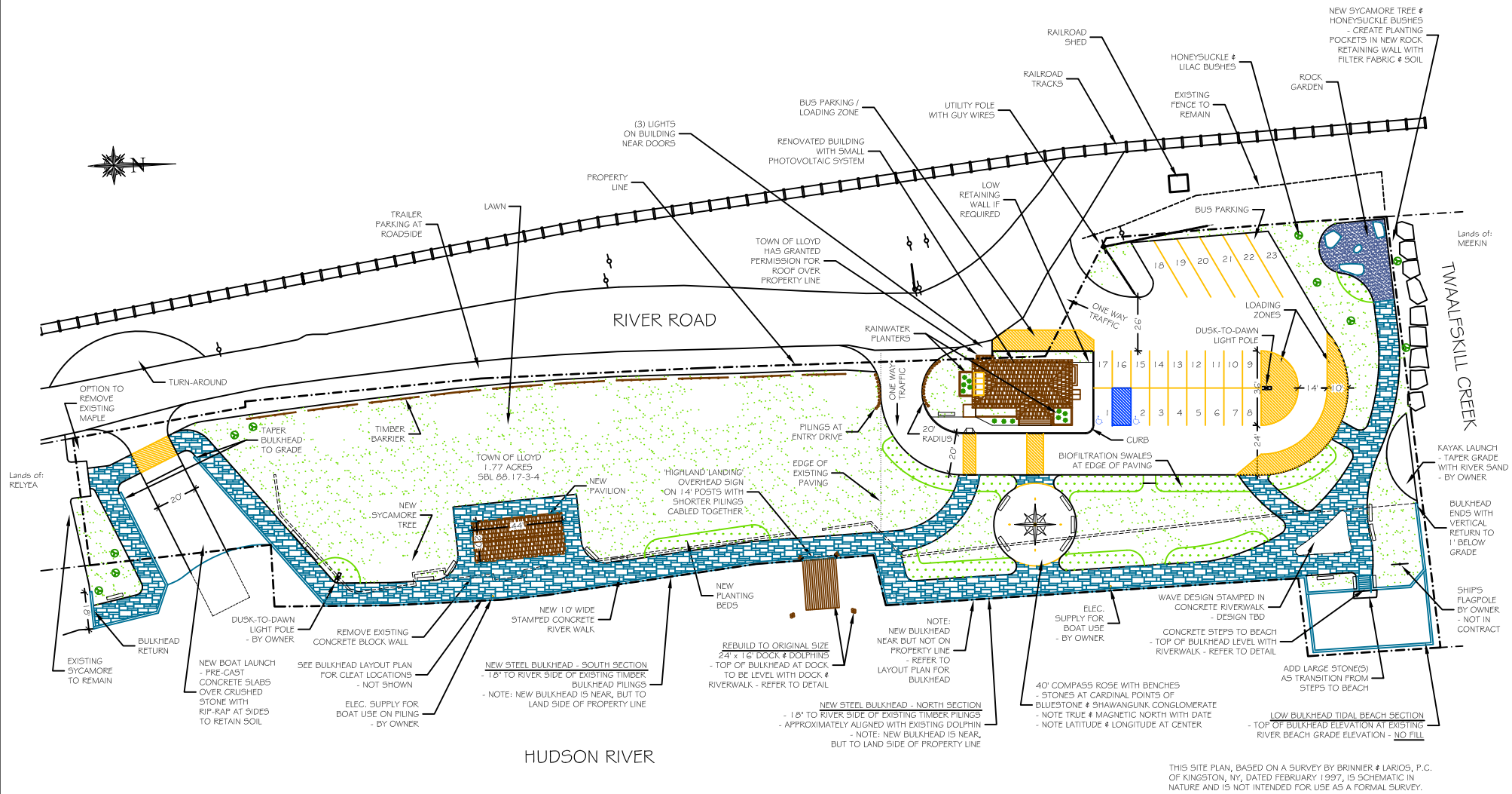
1 SITE PLAN SCALE: 1" = 70'
